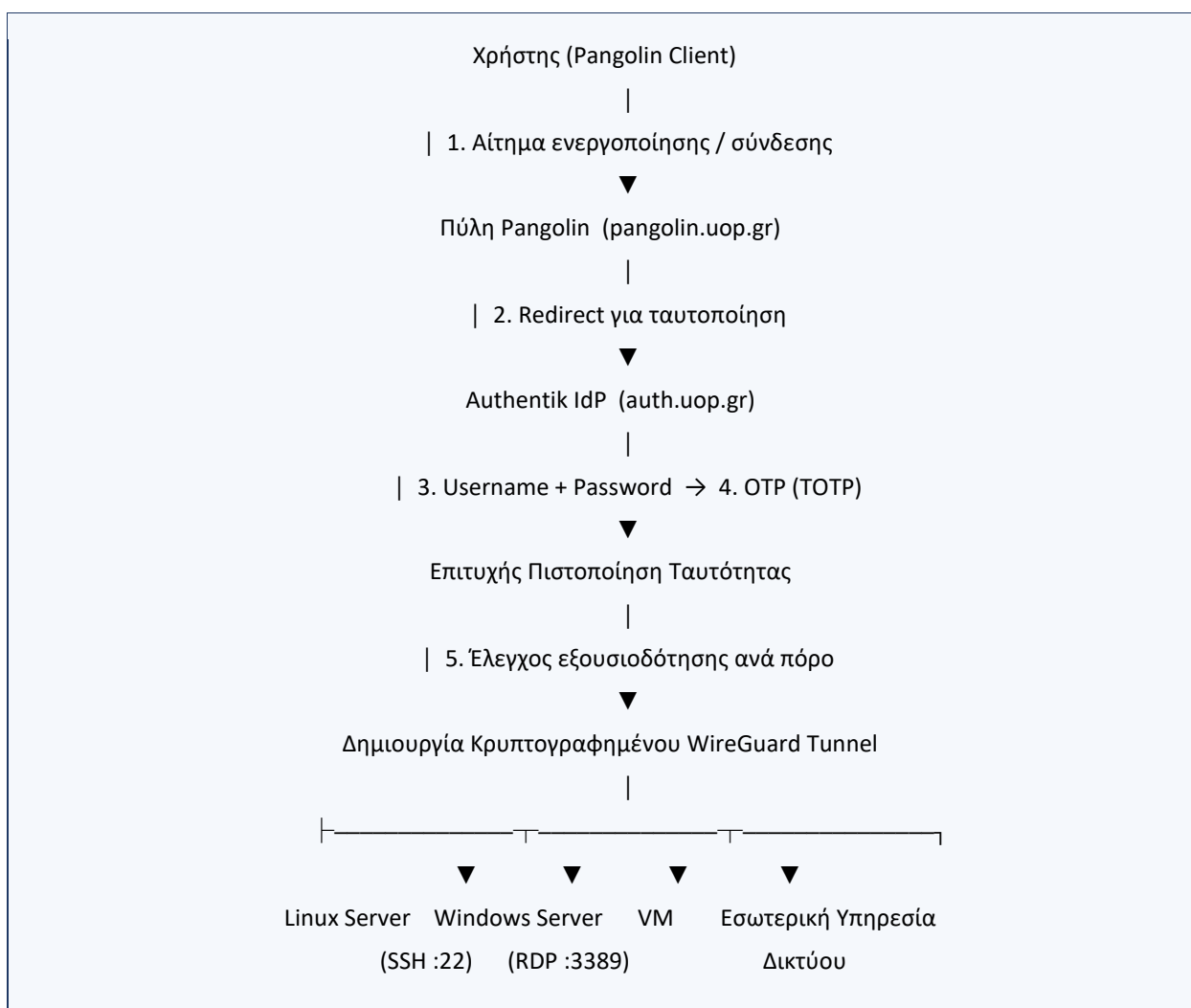
Διάγραμμα 1 — Ροή πιστοποίησης και δημιουργίας ασφαλούς διαύλου πρόσβασης.
